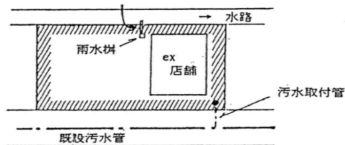
図. エ 単体の開発の場合（店舗や住宅用地等から道路側溝又は水路への排水管）
