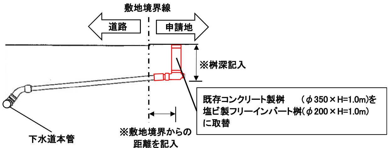
断面図
