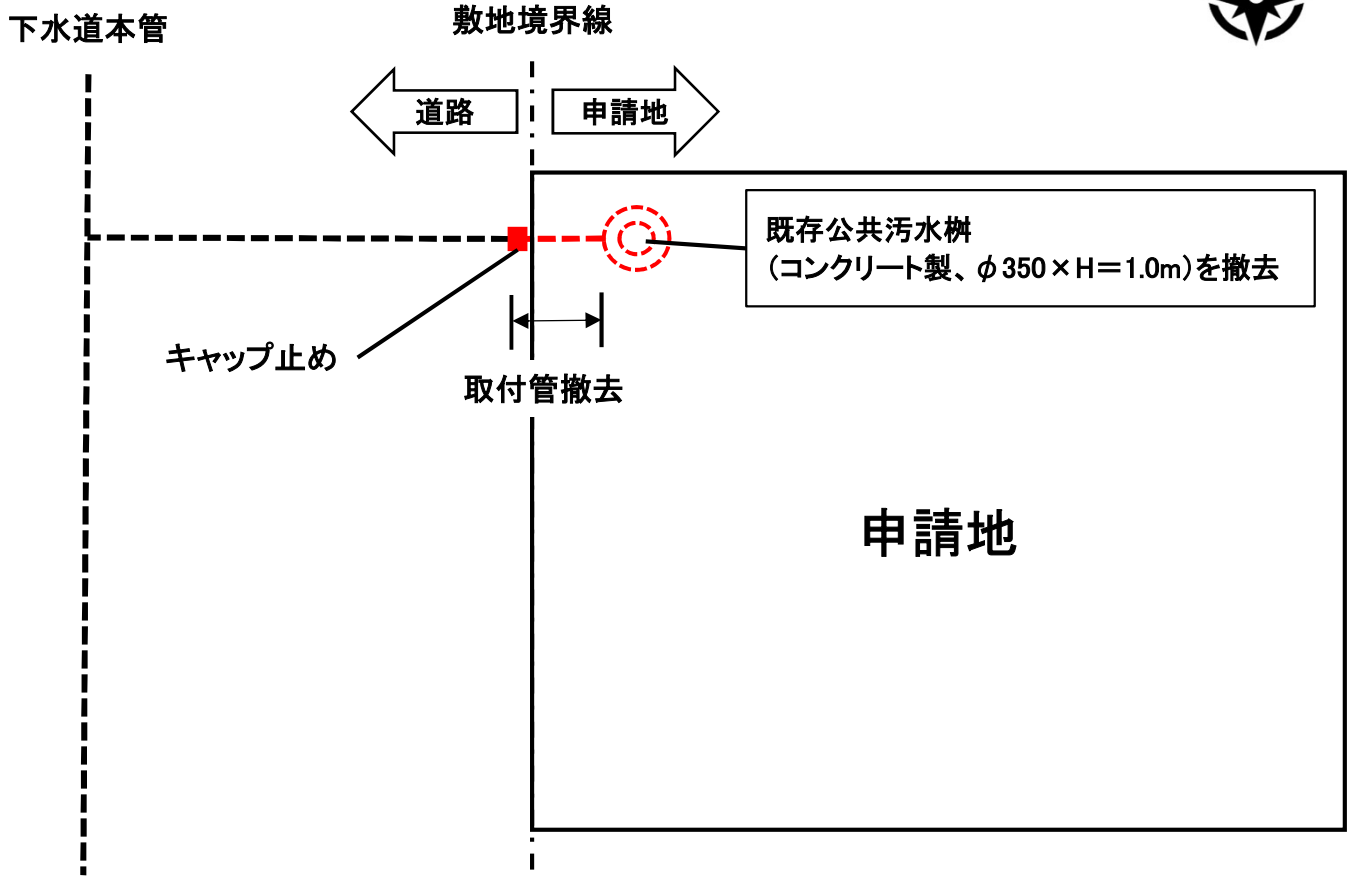
平面図
