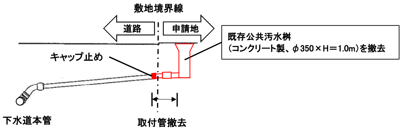
断面図
