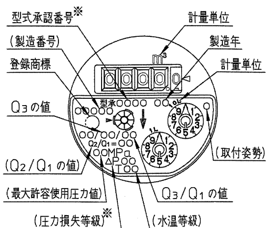
目盛板の例（※は JIS で規定していない項目）
