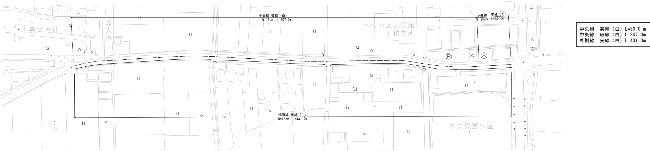
稗田町（高田稗田美濃庄線） 平面図（S=1：1000）
