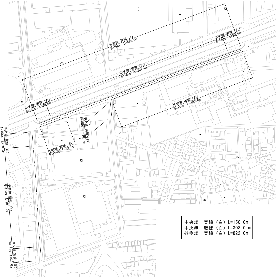
池沢町（昭和工業団地10～1、7～2号線） 平面図（S=1：2000）
