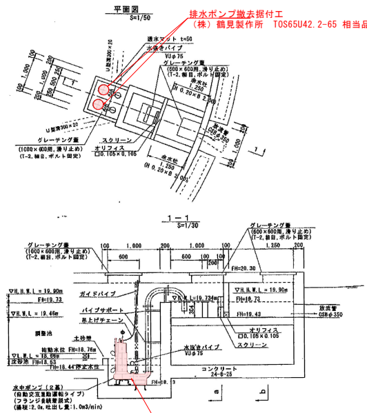
排水ポンプ撤去据付工 (株) 鶴見製作所 TOS65U42.2-65 相当品
