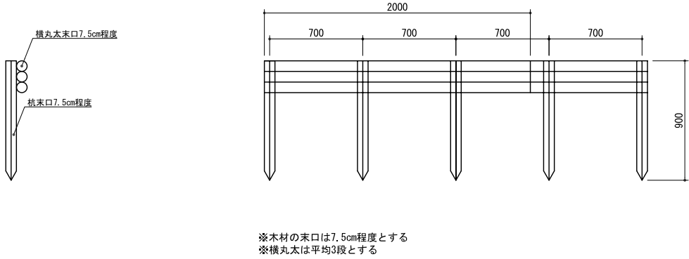
断面図 S=1/20
