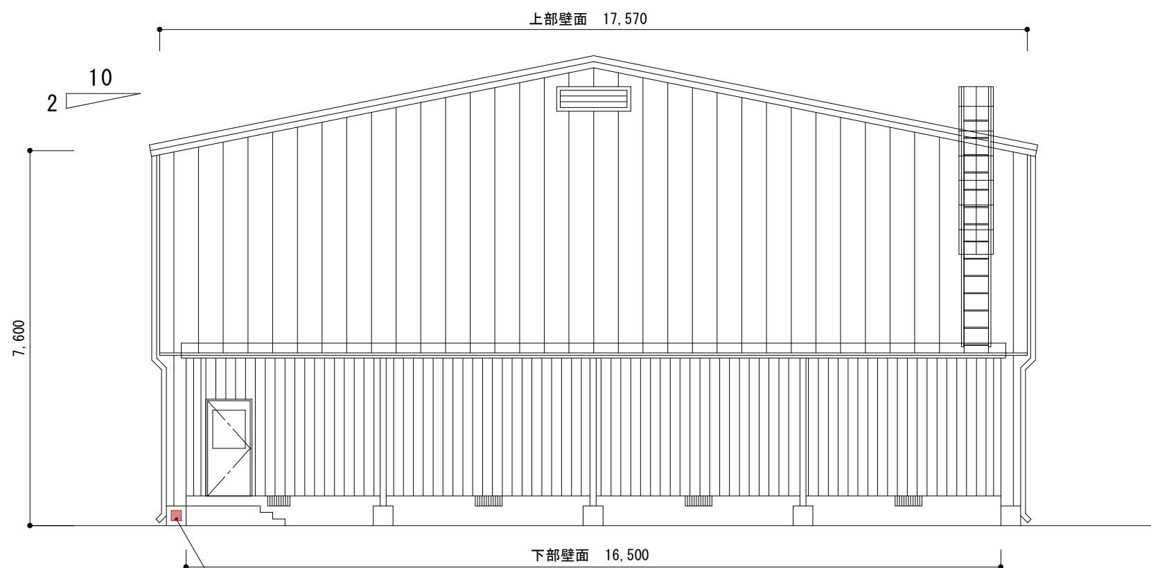
北立面図
