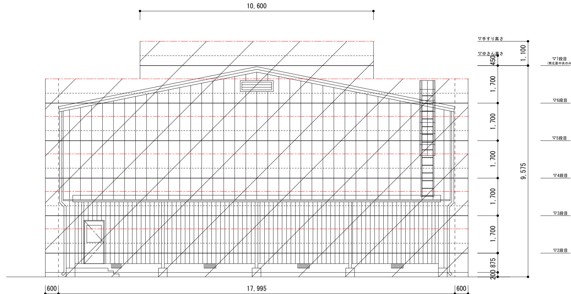
北立面図
