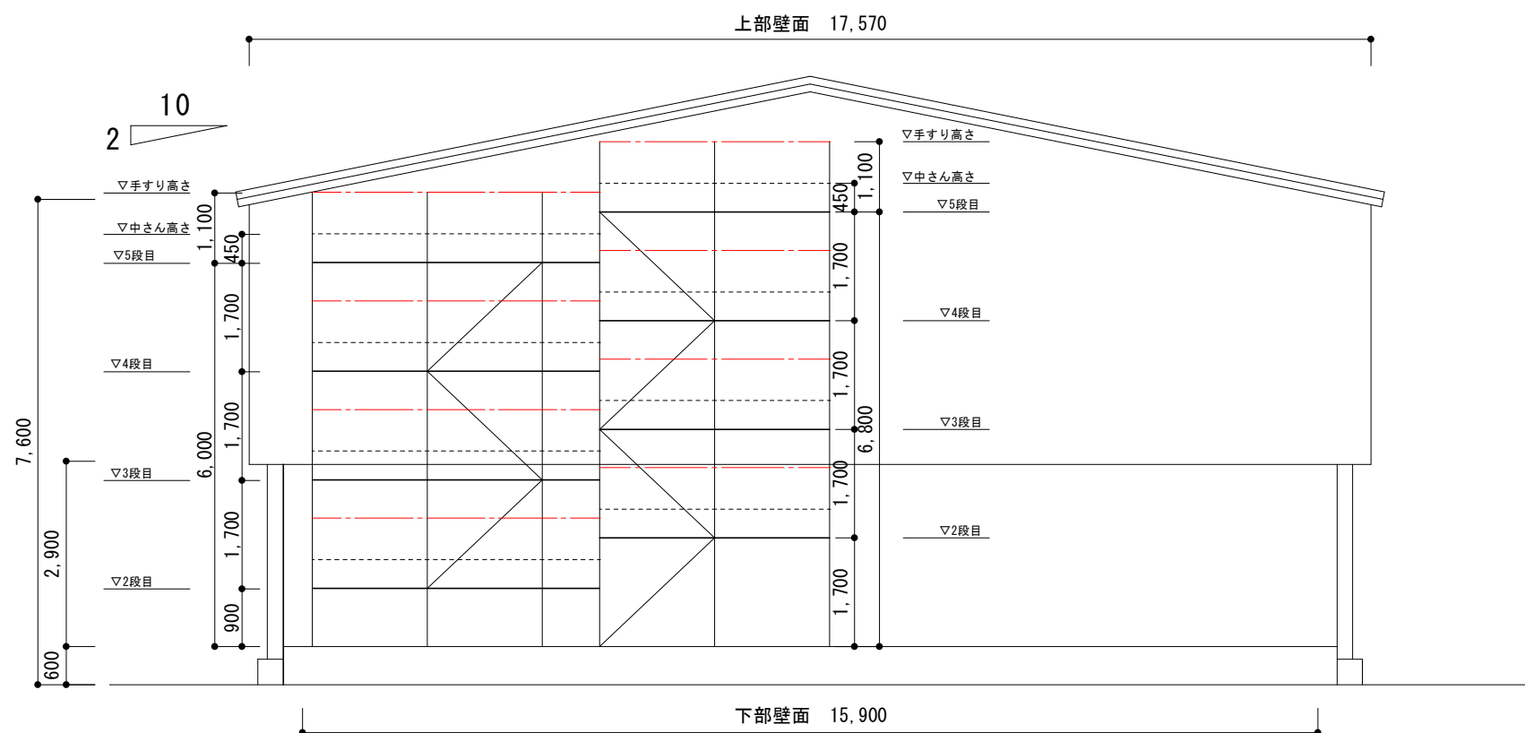
西立面図
