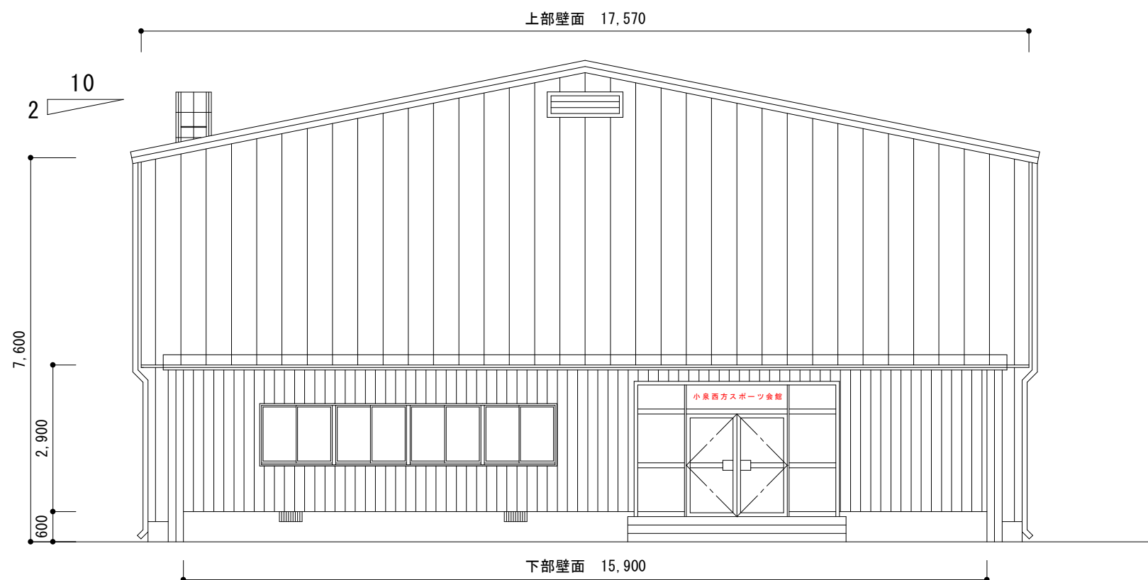
西立面図
