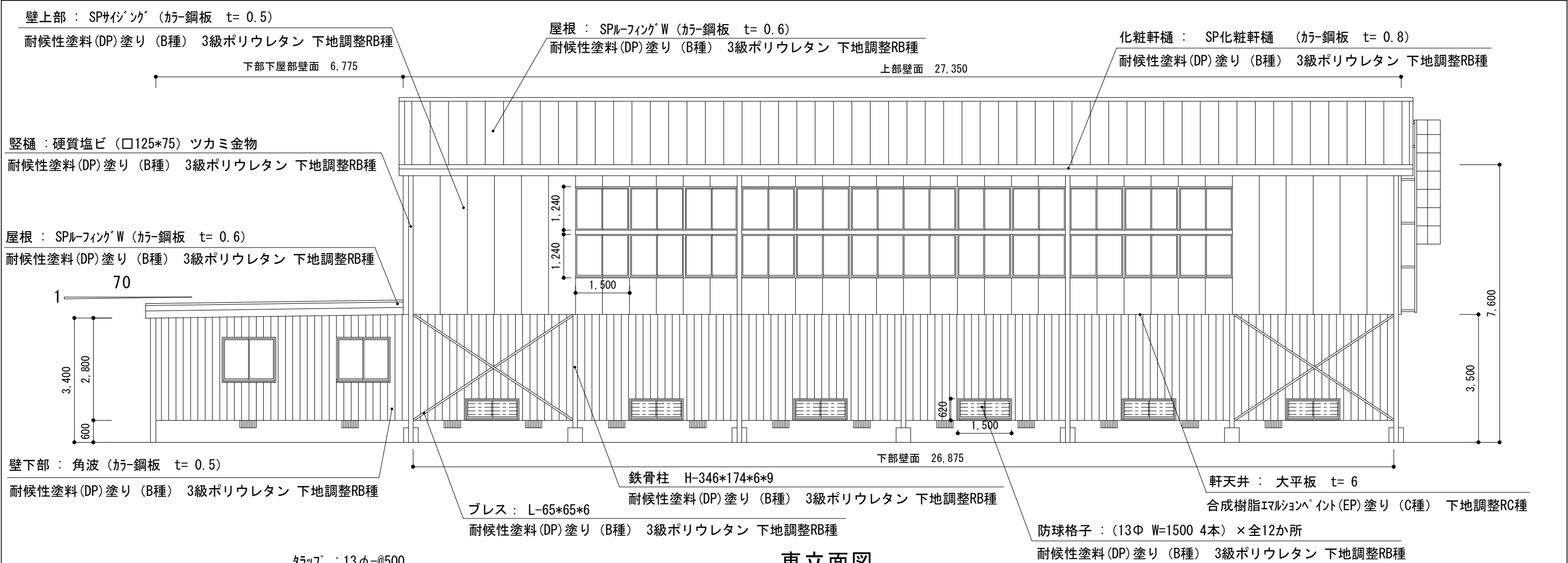
東立面図
