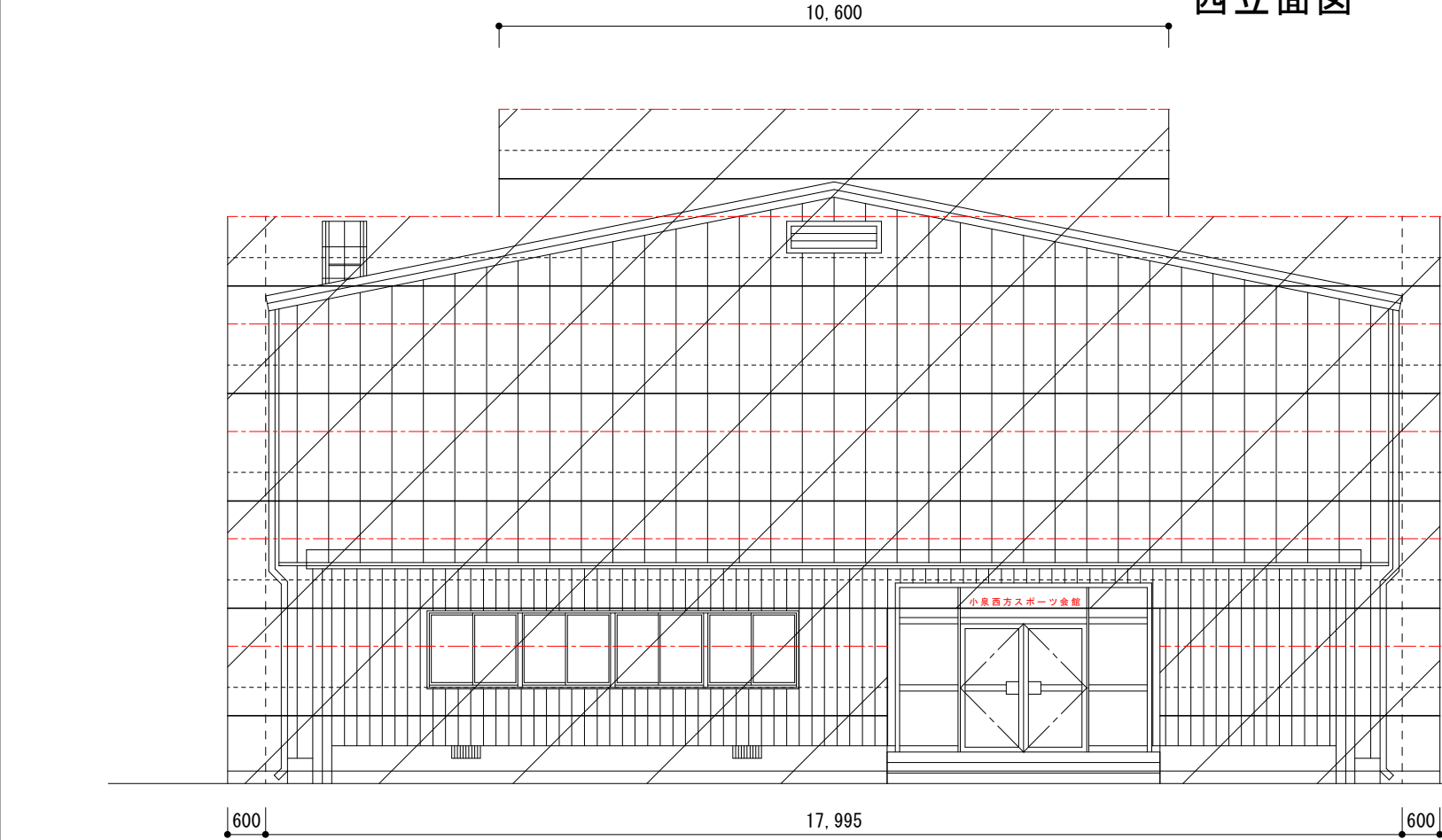
南立面図
