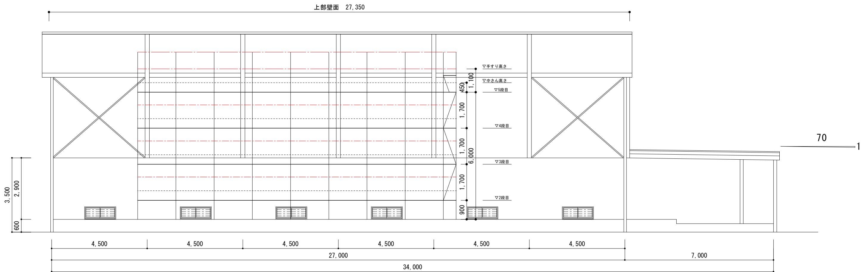
西立面図
