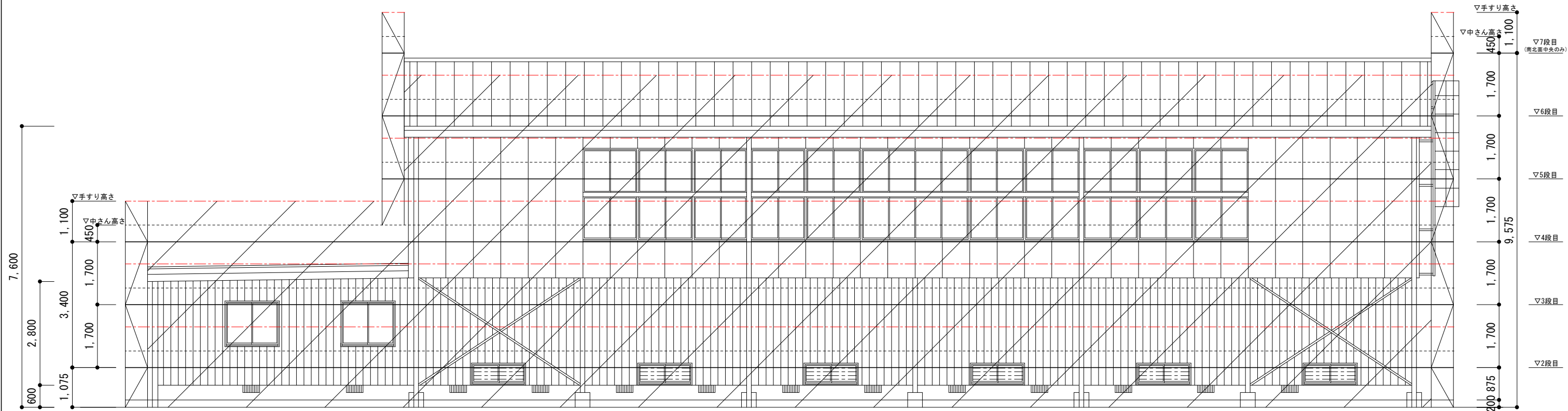
東立面図
