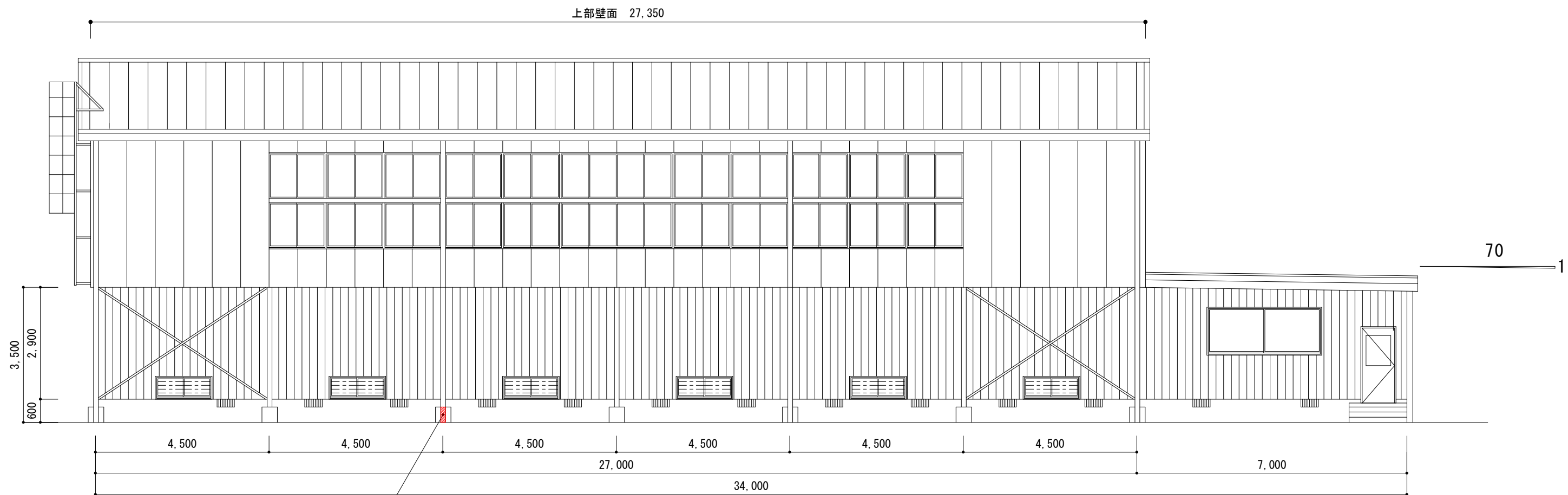
西立面図
