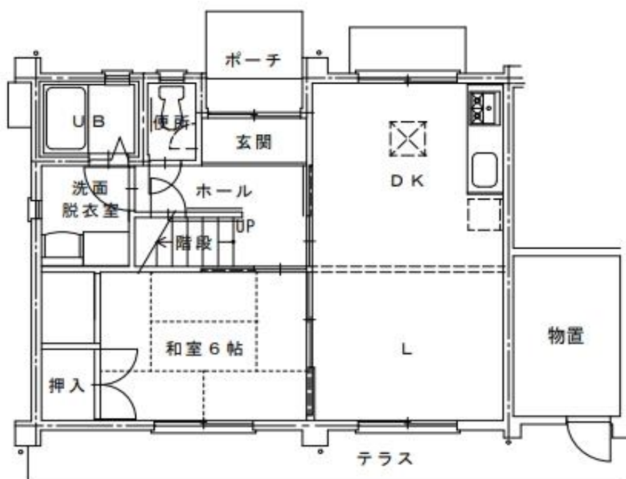
1 階 平 面 図
