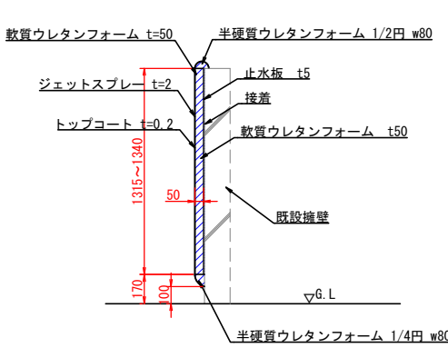
外野 壁面緩衝材断面図 S=1:20
