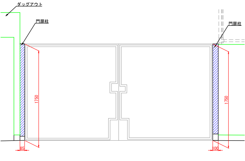
3塁側門扉 壁面緩衝材断面図 S=1:20
