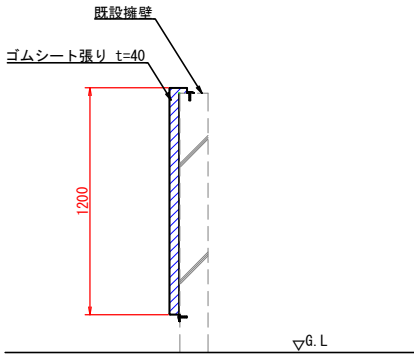
外野 壁面緩衝材断面図 S=1:20
