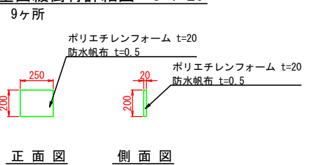
バックネットH型鋼カバー 壁面緩衝材詳細図 S=1:20
