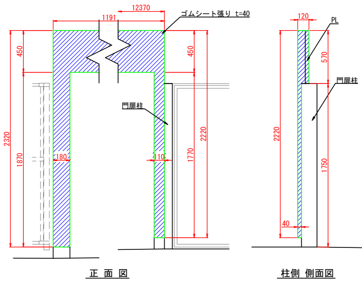
3 塁側ダッグアウト 壁面緩衝材断面図 S=1:20
