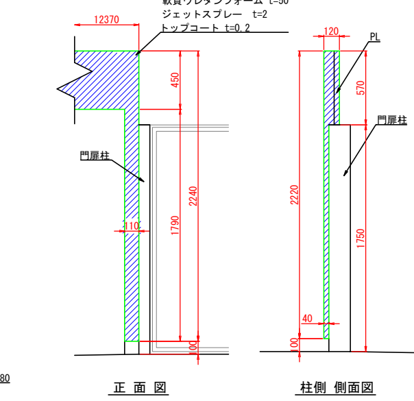
3塁側ダッグアウト 壁面緩衝材断面図 S=1:20
