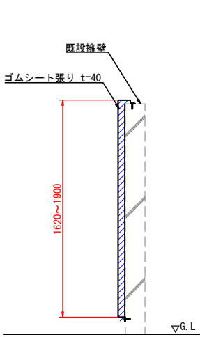
1 塁側 壁面緩衝材断面図 S=1:20
