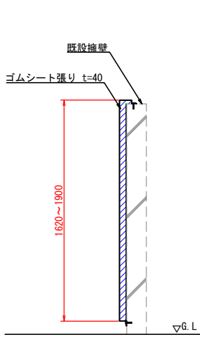
3 塁側 壁面緩衝材断面図 S=1:20
