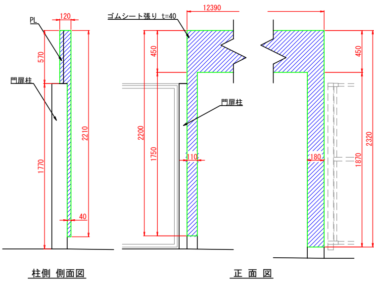
1 塁側ダッグアウト 壁面緩衝材断面図 S=1:20
