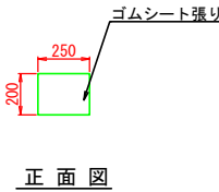
バックネットH型鋼カバー 壁面緩衝材詳細図 S=1:20 9ヶ所
