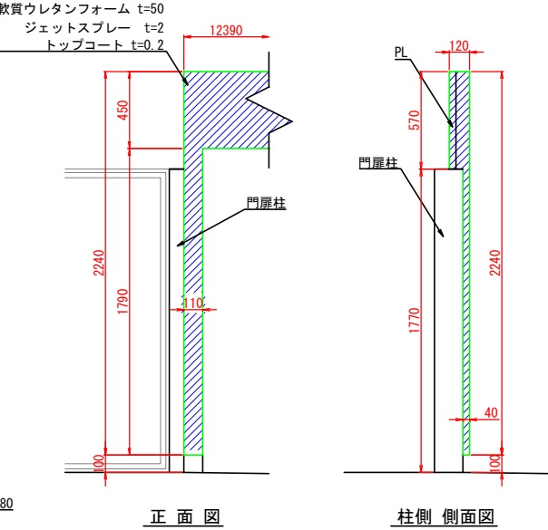
1塁側ダッグアウト 壁面緩衝材断面図 S=1:20
