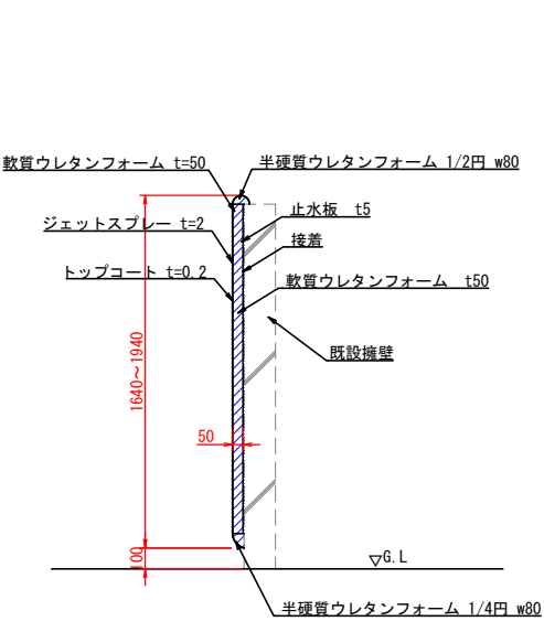
3塁側 壁面緩衝材断面図 S=1:20
