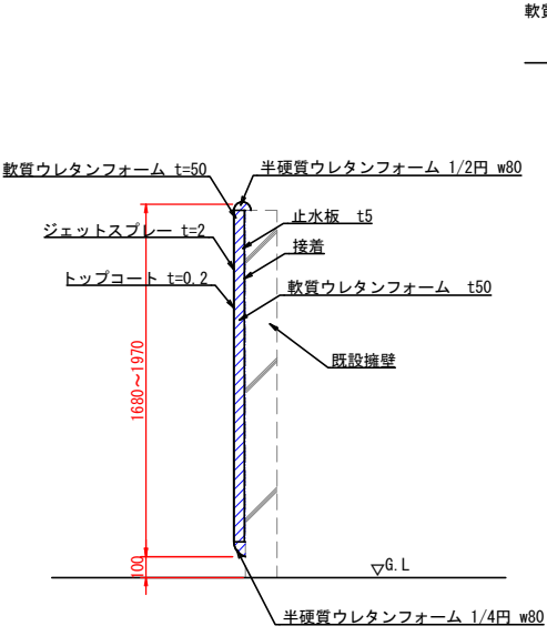
1塁側 壁面緩衝材断面図 S=1:20
