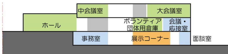
A案 A-A' 断面図
