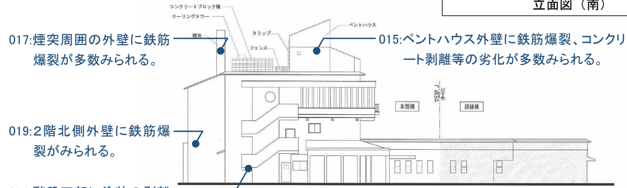
立面図（南）
