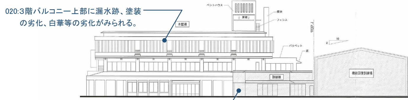
立面図（南）
