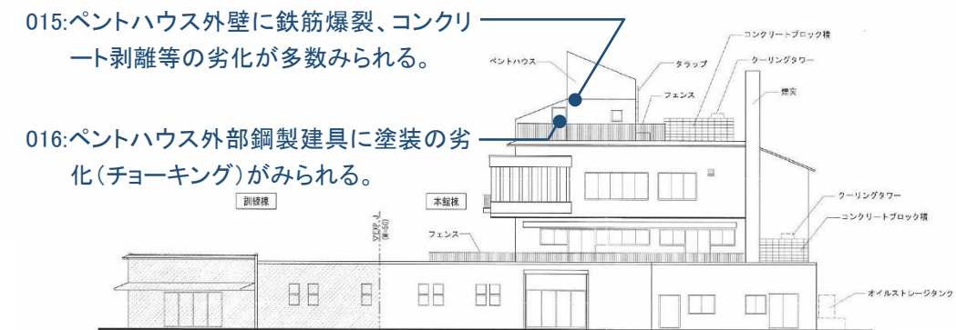
立面図（北）
