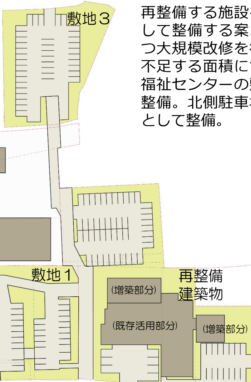
図：再整備計画B案配置図 敷地2
