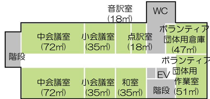
B案 2階ブロックプラン
