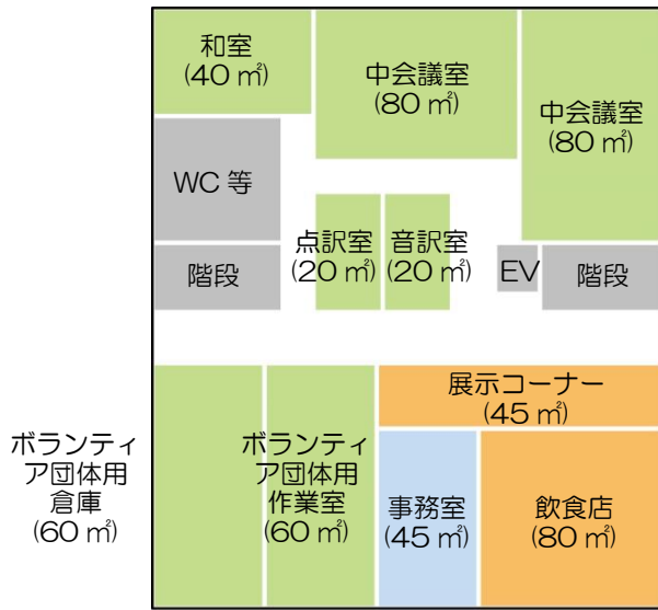
C案 再整備建物1 1階ブロックプラン
