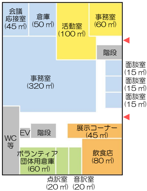
A案 1階ブロックプラン
