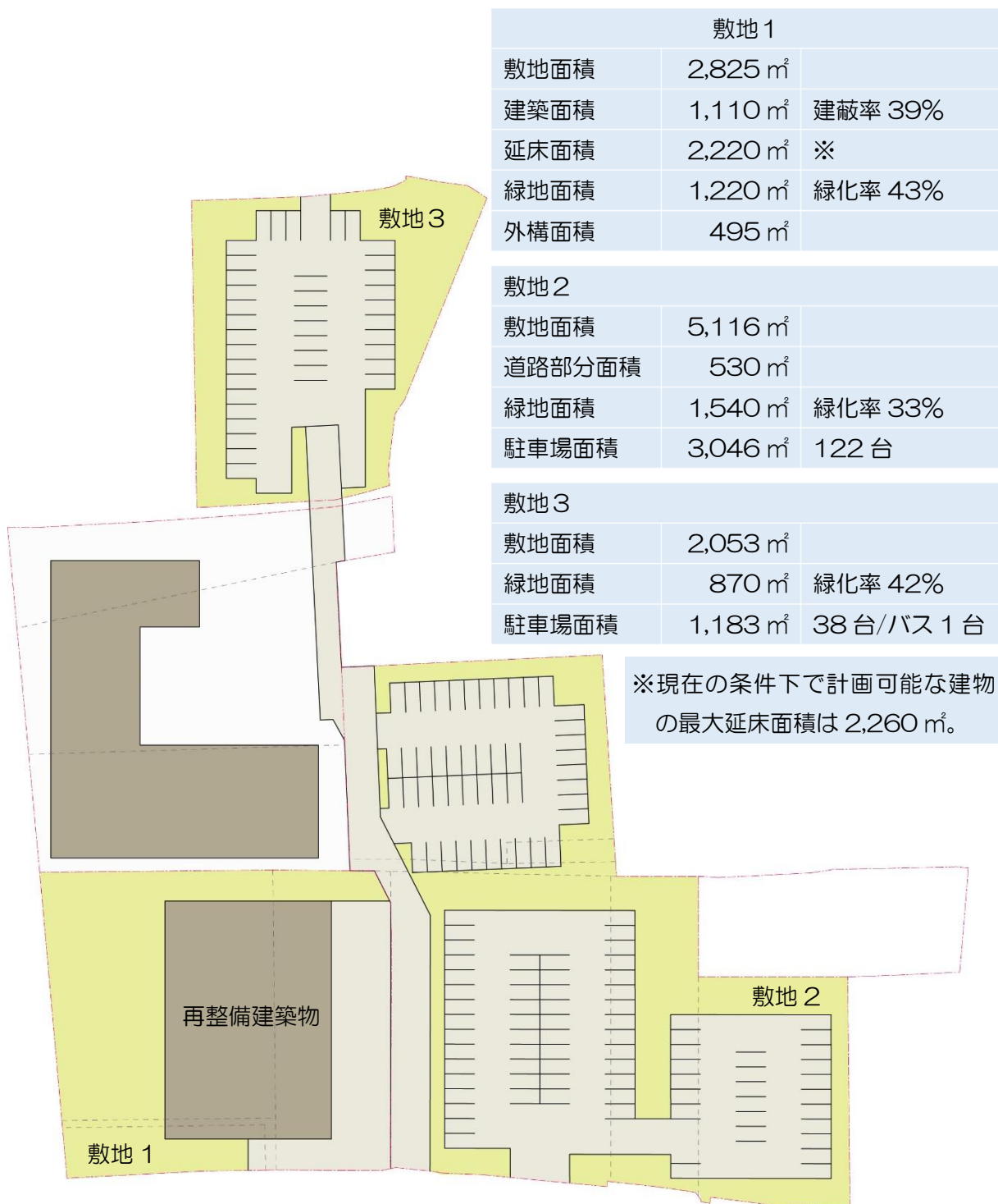
図：再整備計画 A 案配置図
