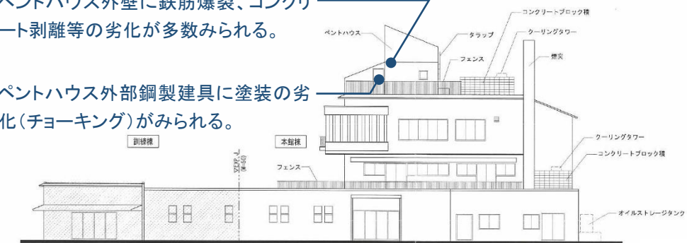
立面図（東）
