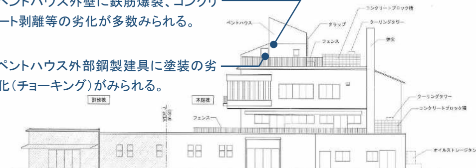
立面図（東）
