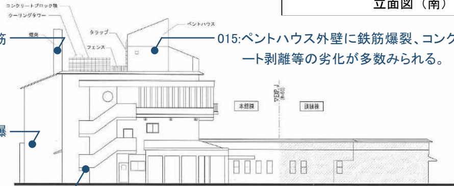
立面図（南）
