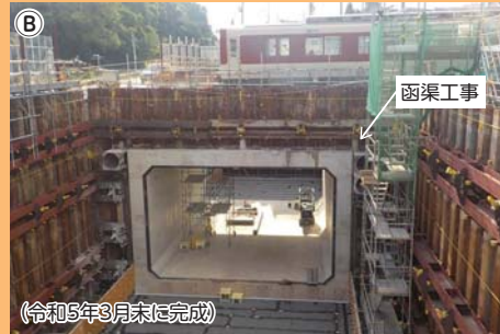
函渠工事(近鉄線路下)
